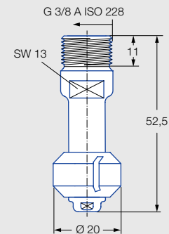
Außengewinde
