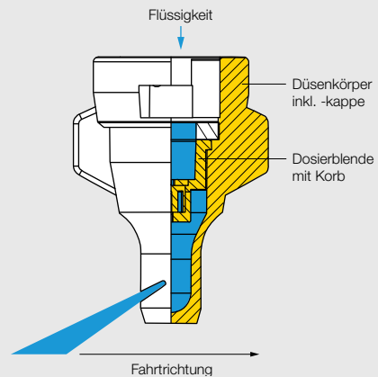
Werkzeuglos herausnehmbare Vorkammer
