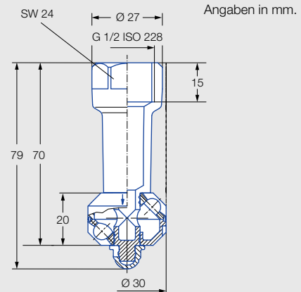
Innengewinde
